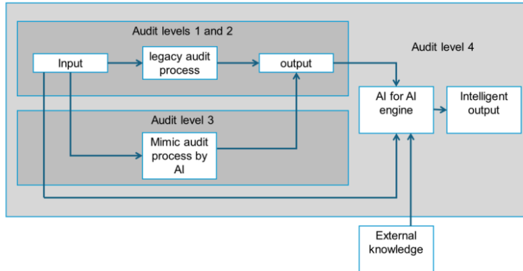
Fig. 4 :- AI for AI process
